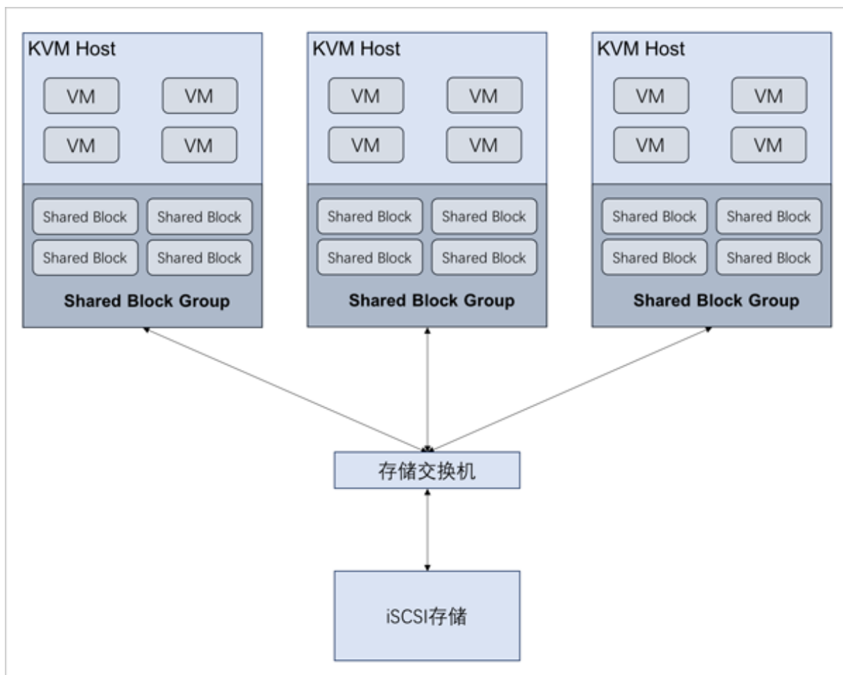
图 1: Shared Block与iSCSI存储网络拓扑图
